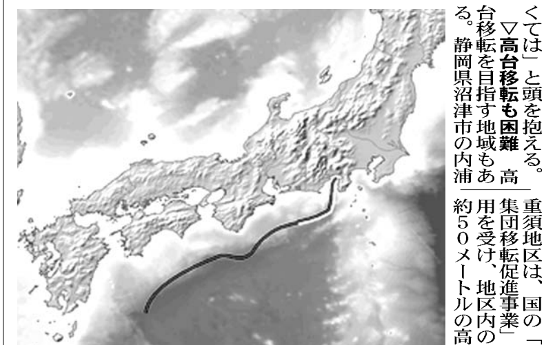
南海トラフの位置(黒線)
