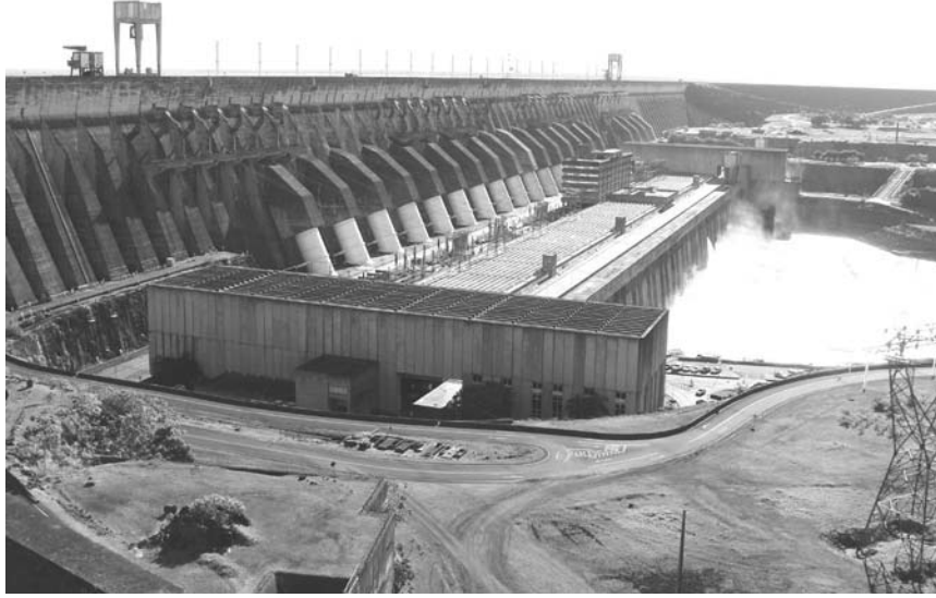
20本(うち2本は保守管理中)のタービンが並び、今も世界一の発電量を誇るイタイプー発電所
