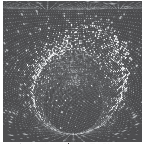
スーパーカミオカンデによる電子型ニュートリノの観測例(東京大宇宙線研究所・T2K提供)
