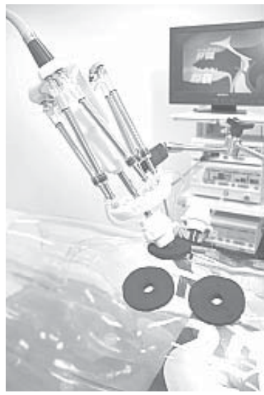
西川教授らが開発した内視鏡手術用ロボット。6本の棒状の装置を挿入してカメラの向きを変える(同教授提供)
