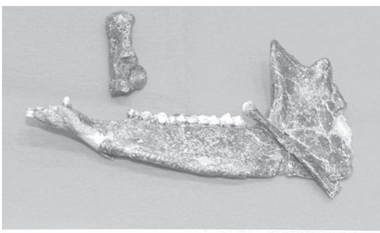
サイの祖先ヒラキウスの下顎(中央)などの化石
