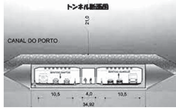
トンネルの断面図
