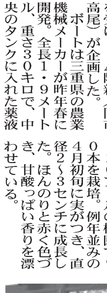
新見市哲西町地区の水田で、ラジコンボートを使った除草剤の散布実演が行われた。写真、高橋が担いだ手不足が進む中、難儀な草取り作業の省力化を求める農家の声を受け、J-A阿新（同市高尾）が企画した。
