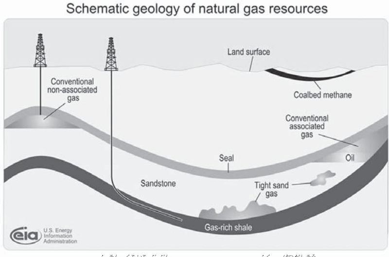
Schematic geology of natural gas resources. シェールガスの賦存(黒色部分)。シェールガスを含む頁岩層 (Gas-rich shale) に水平にパイプを入れ、高水圧で人工的に割れ目をつくり、ガスを採取する。By US Energy Information Administration [Public domain], via Wikimedia Commons
