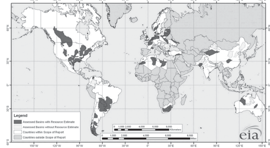
米エネルギー情報局 (EIA) による主なシェールガス層の分布図 (By Energy Information Administration [Public domain], via Wikimedia Commons)
