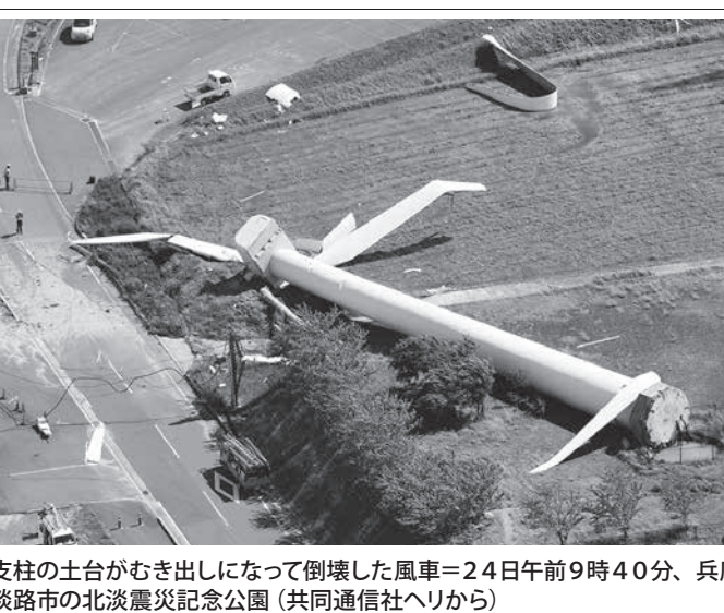
支柱の土台がむき出しになって倒壊した風車=24日午前9時40分、兵庫県淡路市の北淡震災記念公園(共同通信社ヘリから)
